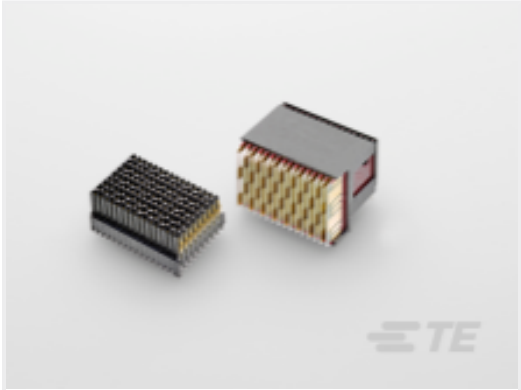
TE 产品编号2302791-1 VERTRECASSY,CENTER,RTM, MULTIGIG RT3
