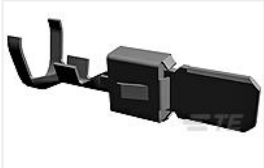
TE 产品编号964310-1 TAB A 5.8x0.8 CONTACT CF SWS Sn
