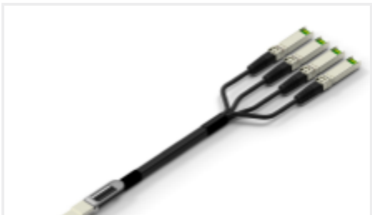
TE 产品编号 CAT-C11-N490333 QSFP28-4 SFP+ 电缆组件：30 AWG
