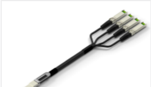
TE 产品编号 CAT-C11-N490325 QSFP28-4 SFP+ 电缆组件：26 AWG
