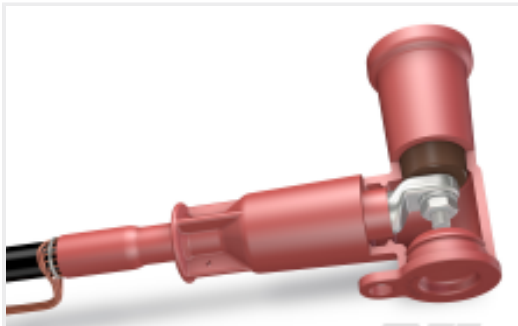
TE 产品编号 CM2361-011 RICS-3133
