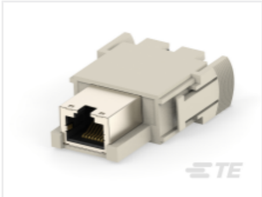
TE 产品编号T2113000201-200 HMN-RJ45-F CAT6A
