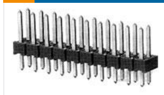
TE 产品编号826632-5 5P AMPMODU II PIN HDR
