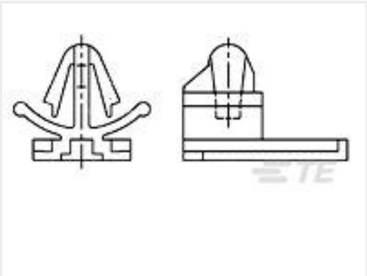
TE 产品编号368165-1 CLIP HSG FOR 070/EJ MK-II(+)
