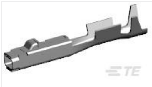
TE 产品编号1670144-1 MCON 1.2 CB REC SRC SN
