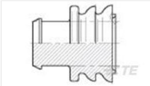
TE 产品编号828986-1 DICHT-STOPFEN
