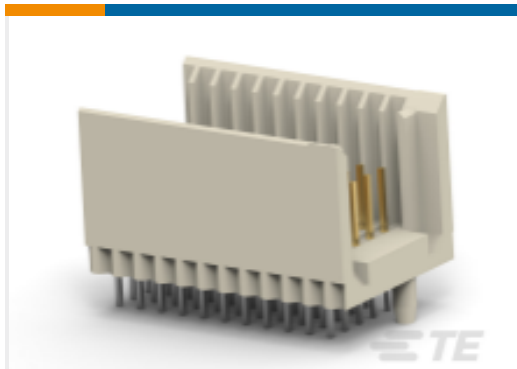
TE 产品编号5352332-1 硬公制公连接器：传统背板，夹层，2mm
