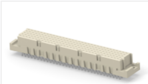
TE 产品编号254123-E STVE 160 F ABCDE VVVV 7-00 EE 4,0 * 247
