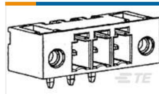
TE 产品编号284541-8 8 POS TERMI-BLOK 900 SF 3,81 m
