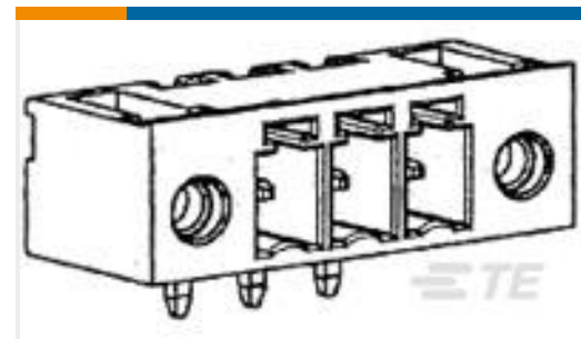
TE 产品编号284541-5 5 POS TERMI-BLOK 900 SF 3,81 m
