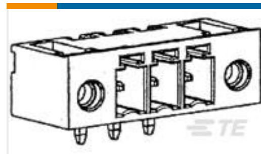
TE 产品编号284541-6 6 POS TERMI-BLOK 900 SF 3,81 m
