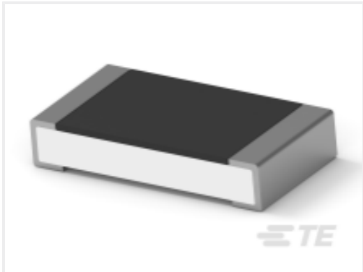
TE 产品编号8-2176391-6 RQ 1206 95K3 0.1% 10PPM 5K RL
