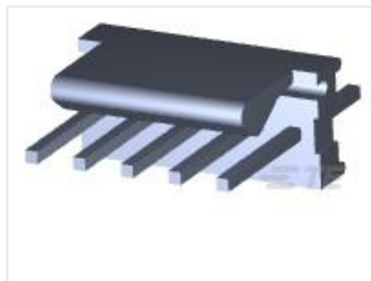
TE 产品编号3-641215-5 05P MTA100 HDR ASSY FL 30AU LF
