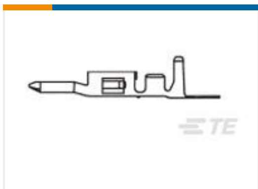
TE 产品编号1586054-1 VAL-U-LOK PIN BR SN 16AWG
