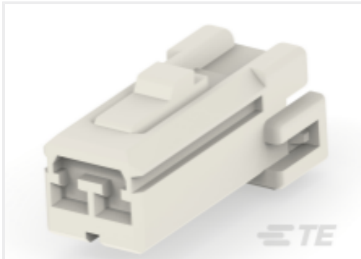
TE 产品编号174463-3 070 MULTILOCK PLUG 2P
