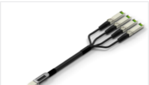
TE 产品编号 CAT-Q17-N49011 QSFP56-4 SFP56 电缆组件：30 AWG
