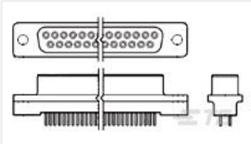
TE 产品编号5745077-3 HD-20 RCPT 15P VERT FFSCRLK
