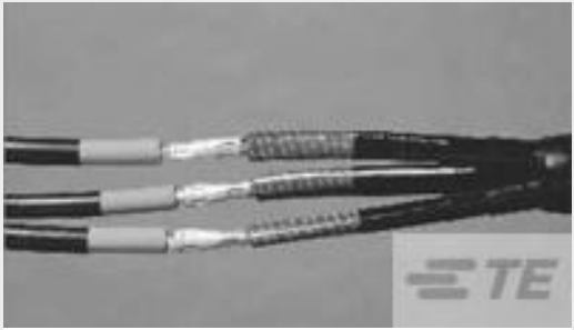
TE 产品编号440655-000 HVS-T-2582E
