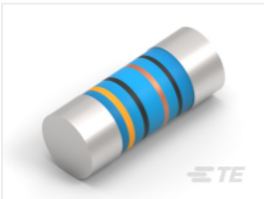
TE 产品编号4-2176315-4 MELF SMA_A 330R 1% 50PPM 0204 0.4W
