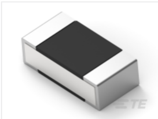
TE 产品编号7-2176307-7 RP 1E 0.1W 76K8 0.1% 25PPM 5K RL
