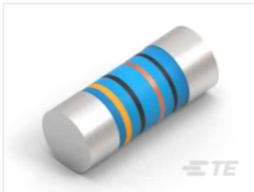
TE 产品编号4-2176315-9 MELF SMA_A 820R 1% 50PPM 0204 0.4W
