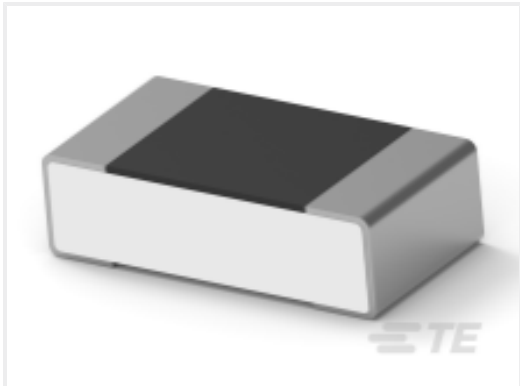
TE 产品编号6-2176366-5 RQ 0603 2K0 0.1% 10PPM 1K RL
