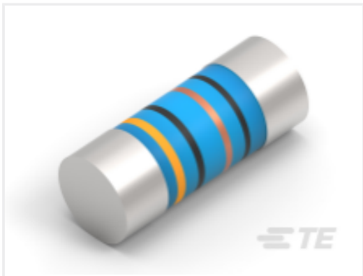
TE 产品编号8-2176314-1 MELF SMA-A 68K 1% 50PPM 0102 0.3 W
