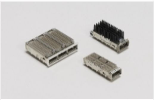
QSFP、QSFP+ 和 zQSPF+(145)
