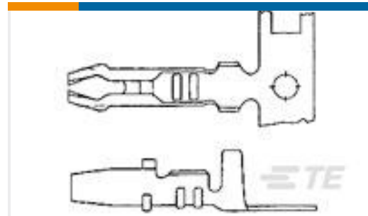
TE 产品编号170072-1 AMP-IN 24-20 AWG
