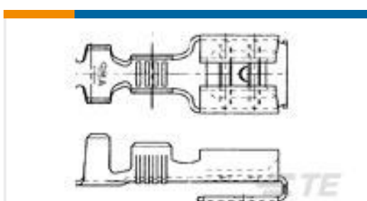
TE 产品编号282349-1 PL 250 FLAG REC 0.5-1.5MM2 0.4 X 44 NISI
