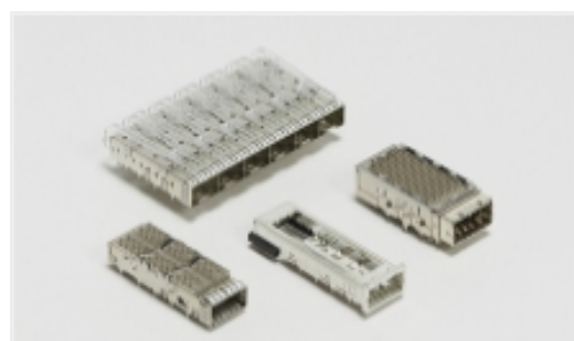
插拔式 IO 连接器和笼子(145)
