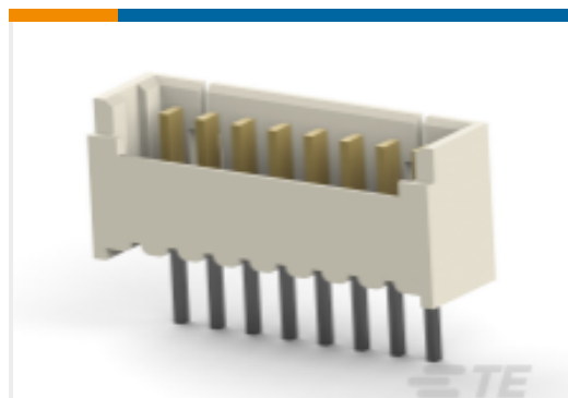
TE 产品编号6-1734598-1 1.25 WTB HDR DIP, L=2.3, 8 POS
