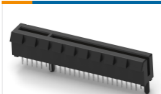
TE 产品编号2-2041242-1 30PCI-E CARD EDGE, 98 POS, 30U",
