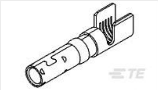
TE 产品编号213843-1 POWERBAND CONT ASSY,SILVER PLT
