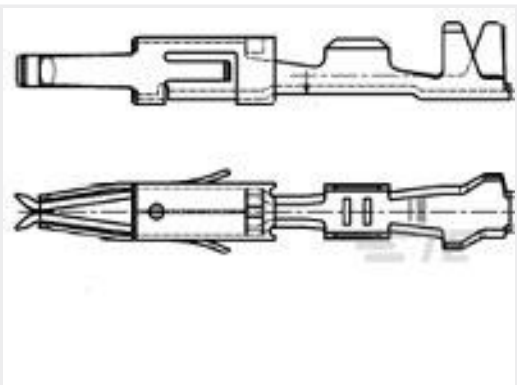
TE 产品编号962875-1 MT2 REC 1.6 Contact SWS Sn
