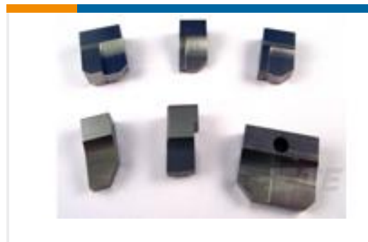
TE 产品编号7-1333201-4 ANVIL, COMBINATION .055
