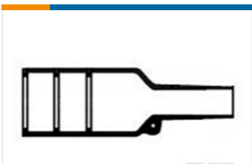
TE 产品编号154665-000 球形热缩护套：有嘴，直形
