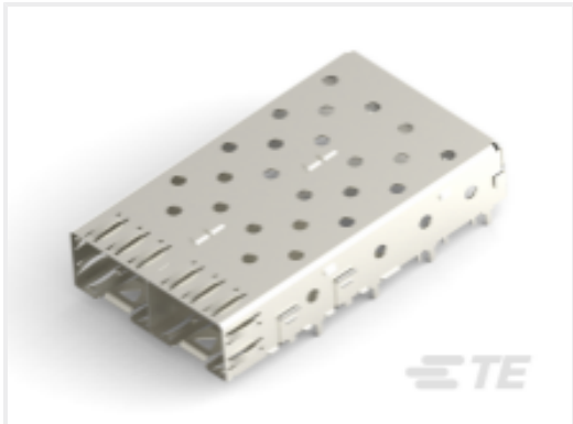
TE 产品编号1761014-3 SFP 1X2 CAGE ASSY, PRESS FIT
