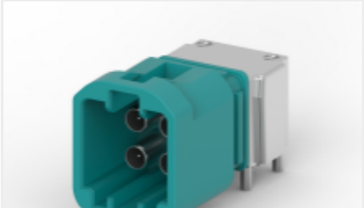
TE 产品编号2304168-9 4P MATE-AX, HDR ASSY,90 DEG,COD Z
