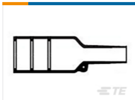
TE 产品编号154665-000 球形热缩护套：有嘴，直形
