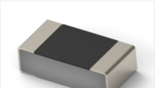
TE 产品编号1676390-2 RN 0805 5K76 0.1% 10PPM 1KRL
