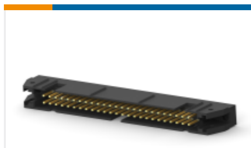
TE 产品编号5499141-4 AMP 锁门通用插头
