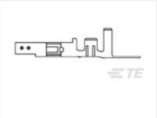
TE 产品编号2238019-1 VAL-U-LOK SKT BR SN 22-26AWG
