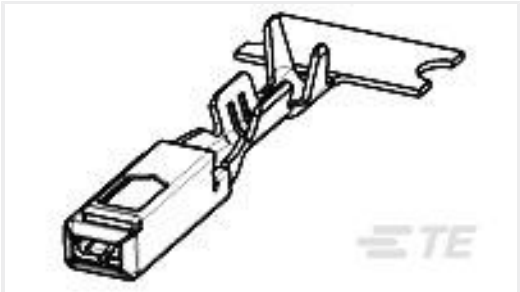
TE 产品编号5-1534116-1 MQS0,63 SN REC CB UNSEAL. 0,25- 0,35 2P
