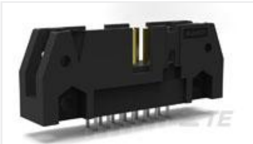
TE 产品编号5102153-8 A/L UNIV HDR 34P VERT
