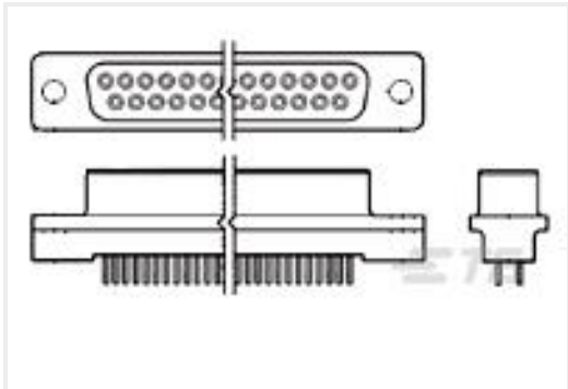
TE 产品编号5207828-4 HD-20 RCPT 25P VERT
