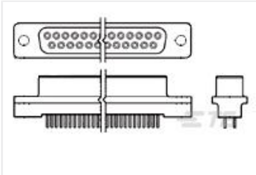
TE 产品编号5207841-3 HD-20 RCPT 9P VERT THD INS
