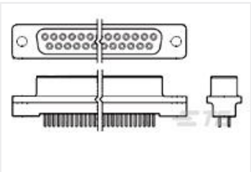
TE 产品编号5207829-4 HD-20 RCPT 37P VERT
