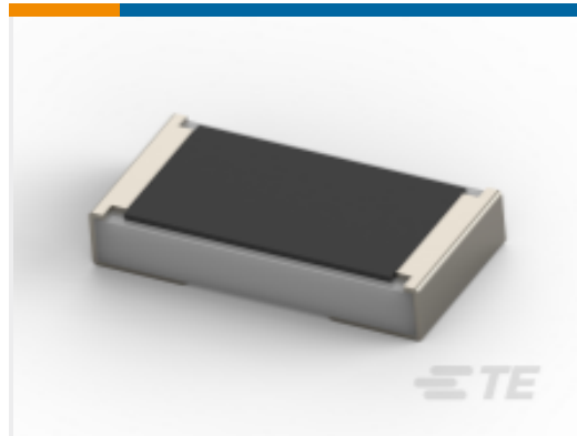
TE 产品编号8-2176231-8 SMD 功率电阻器 : 3 瓦特 , 1% Tol
