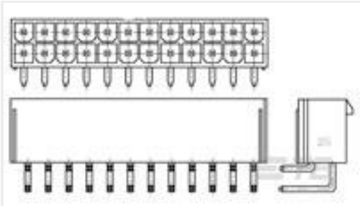
TE 产品编号1586041-2 2P VAL-U-LOK R/A HDR V2
