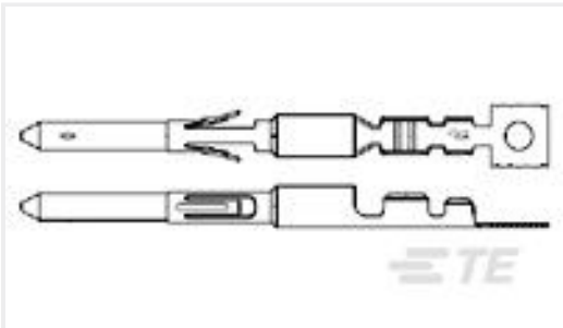
TE 产品编号66735-2 DIN CONN PIN CONT
