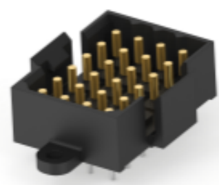
TE 产品编号 1-206763-3 METRIMATE PIN HEADER ASSY,24P
