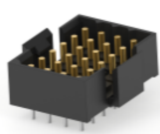
TE 产品编号 1-206763-4 METRIMATE PIN HDR ASSY,24P LF
