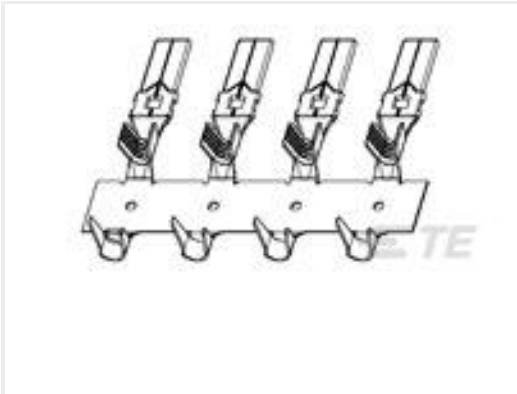
TE 产品编号1670225-1 TAB 6.3 X 0.8 BODY BUSBAR
