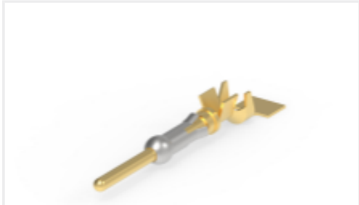
TE 产品编号 1-66597-1 III+ PIN,18-14,TIN ,STRIP
