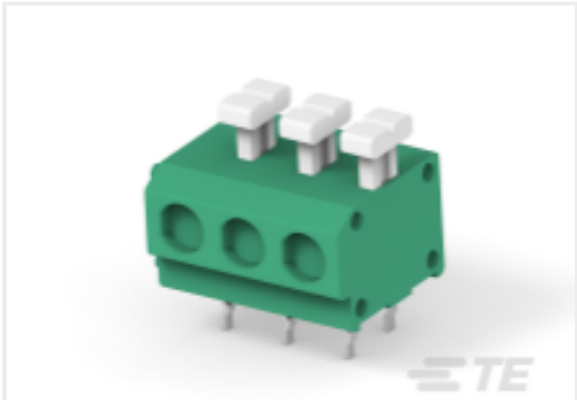
TE 产品编号1-2834018-3 3POS 5.0MM TEPS CONN.
