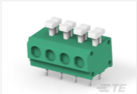
TE 产品编号1-2834018-4 4POS 5.0MM TEPS CONN.
