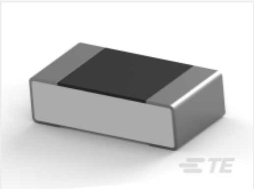
TE 产品编号3-2176370-3 RQ 0603 931R 0.1% 10PPM 5K RL
