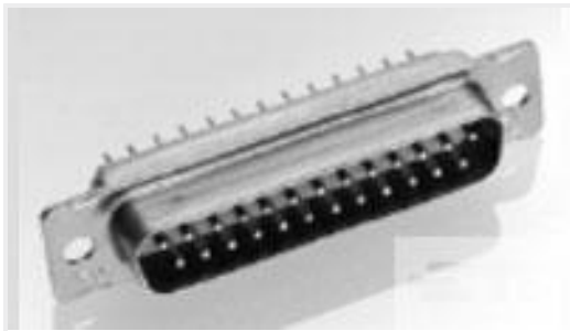
TE 产品编号 204503-1 AMPLIMITE,ASY,PLUG,STD,90,2
