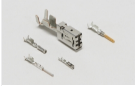
汽车端子(43)
