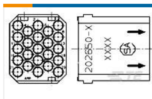
TE 产品编号202650-4 PIN MODULE, 23 POSN, G-SERIES
